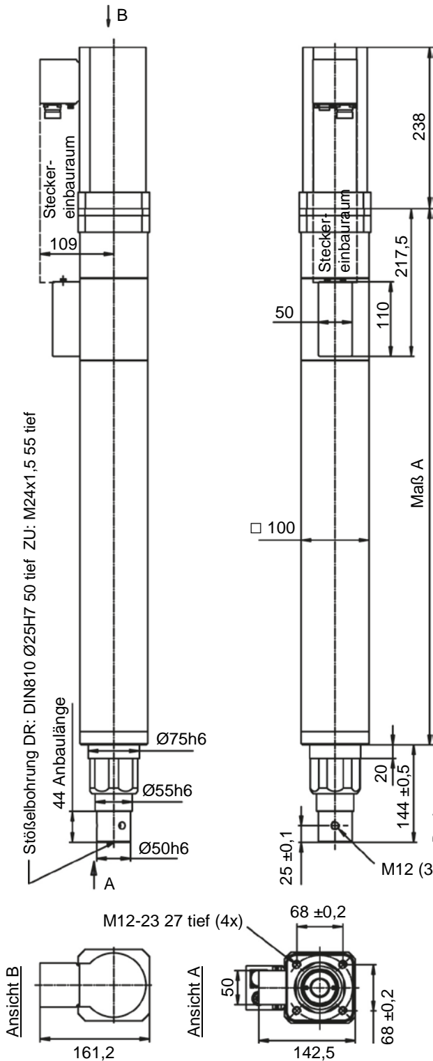
QMP 100 /30/40/50 Motor stehend
