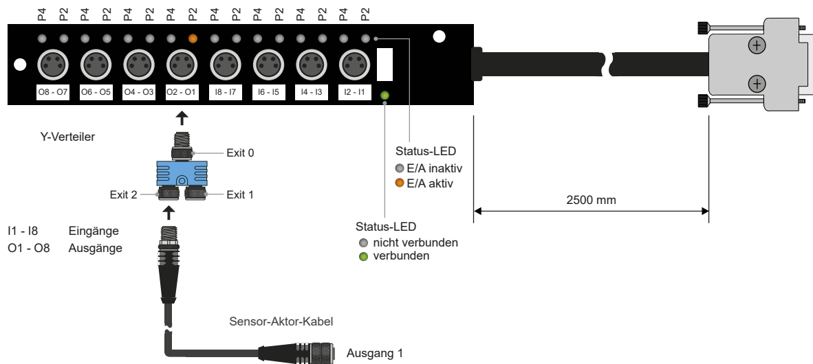
E/A-Expander 8/8 (8 Ports, Dual) inkl. Kabel (MS-1002208)
